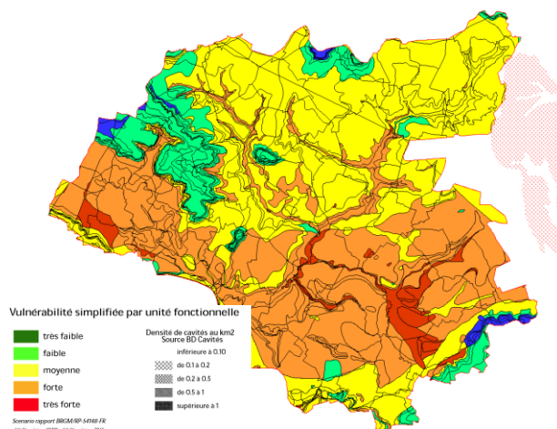
Vulnérabilité intrinsèque des nappes souterraines
